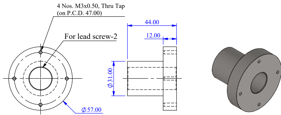
DETAILS OF NUT-2 MATERIAL: DELRIN QTY.- 1 no.
